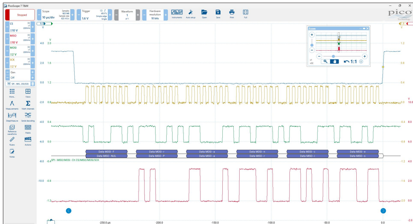
SPI 接口
